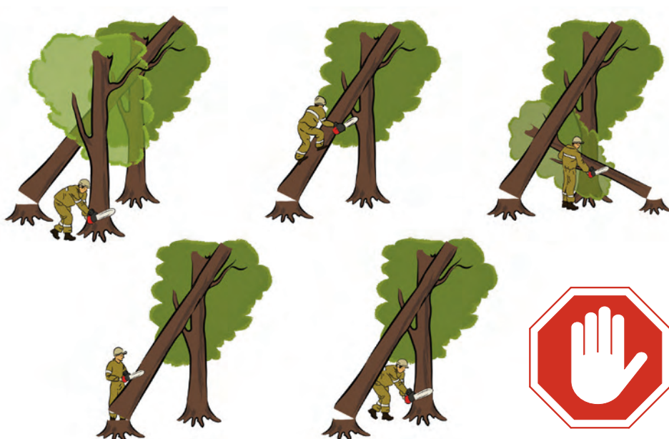
Рис. 46. Запрещённые методы валки зависших деревьев. Автор: Елена Ефремова
