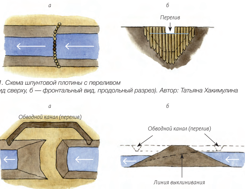
Рис. 32. Схема торфяной плотины с переливом (а — вид сверху, б — вид сбоку, поперечный разрез). Автор: Татьяна Хакимулина
